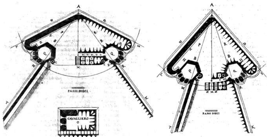
Figura 31 – Geometria das cidadelas (II)
