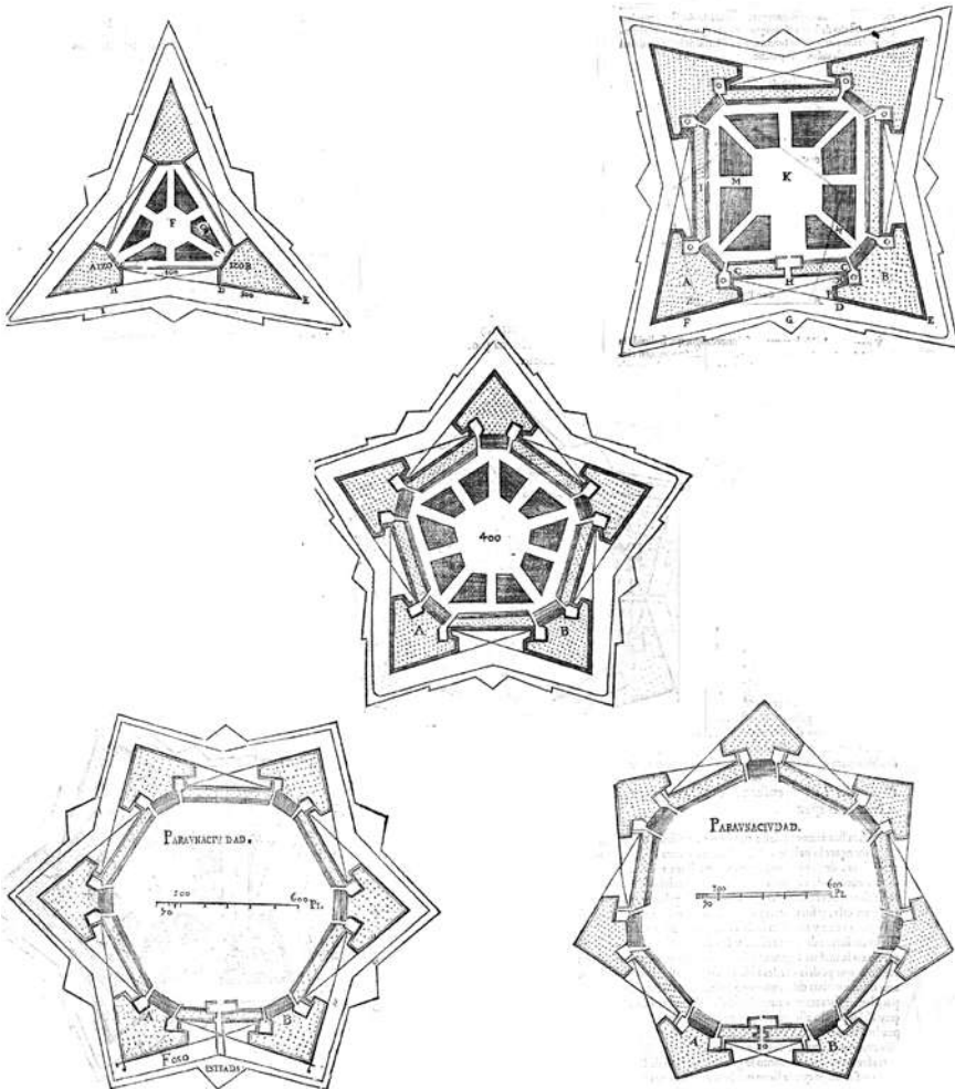
Figura 30 – Geometria das cidadelas (I)
