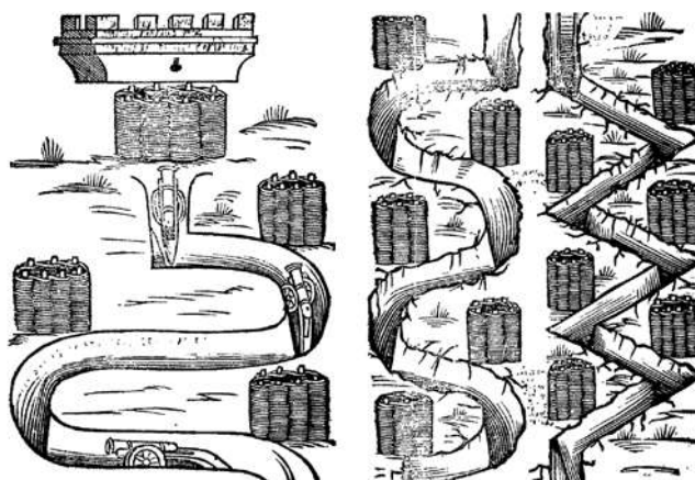
Figura 173 – Fortificações de assédio (I)
